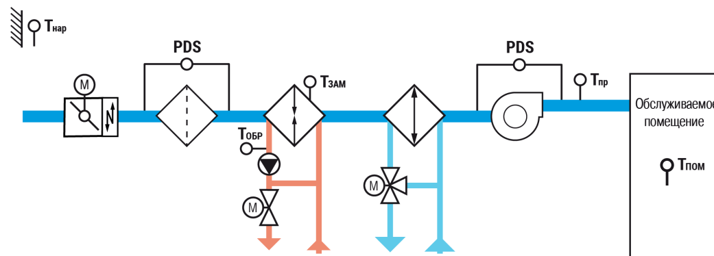
Рисунок 6.5 – Функциональная схема установки
