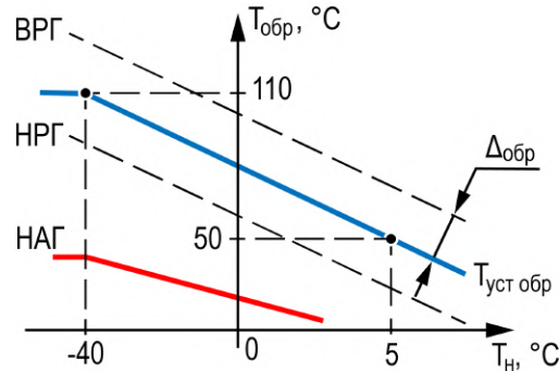
Рисунок 10.11 – График T_{обр}(T_n)
