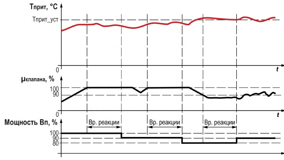
Рисунок 10.10 – Иллюстрация работы функции снижения производительности вентилятора при нехватке мощности нагрева
