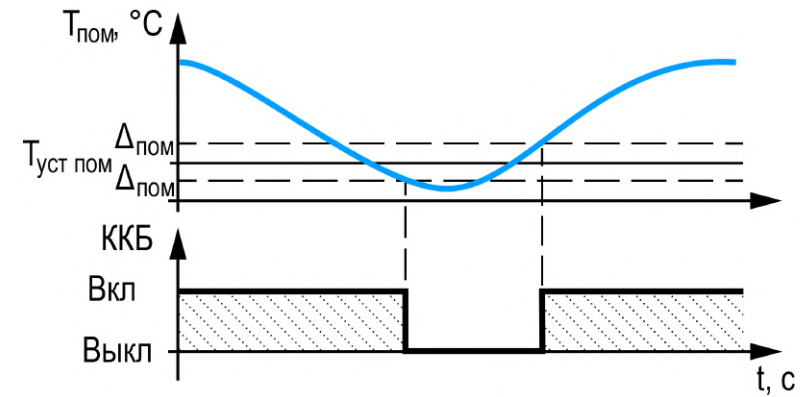
Рисунок 10.21 – Управление ККБ
