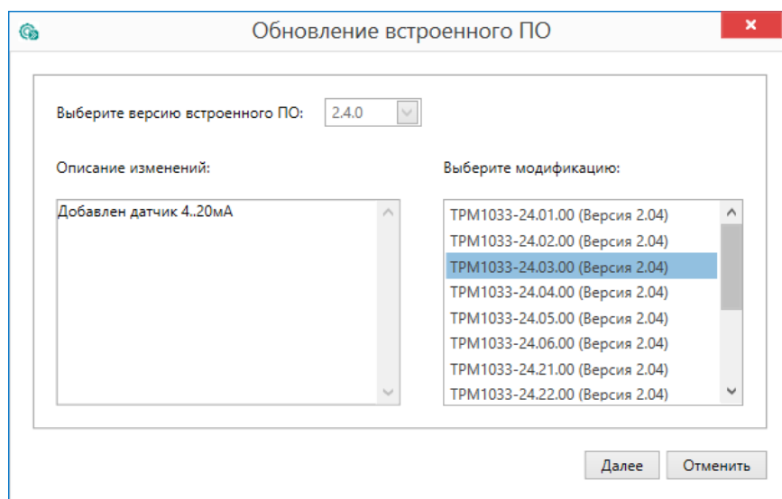
Рисунок 11.7 – Выбор алгоритма
